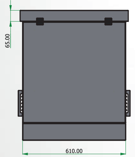
ARKA GÖRÜNÜŞ
