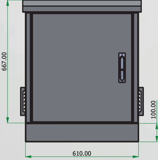
ÖN GÖRÜNÜŞ
