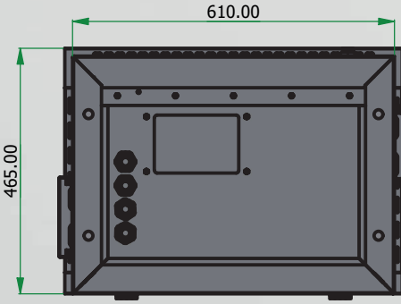
ALT GÖRÜNÜŞ
